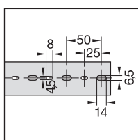
Perforation du fond DIN 43659 EN 50 085-2-3 largeur 25, 40 et 60 mm
