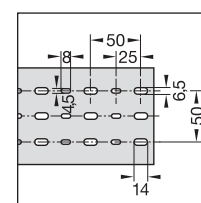
Perforation du fond DIN 43659 EN 50 085-2-3 largeur 80, 100 et 120 mm
